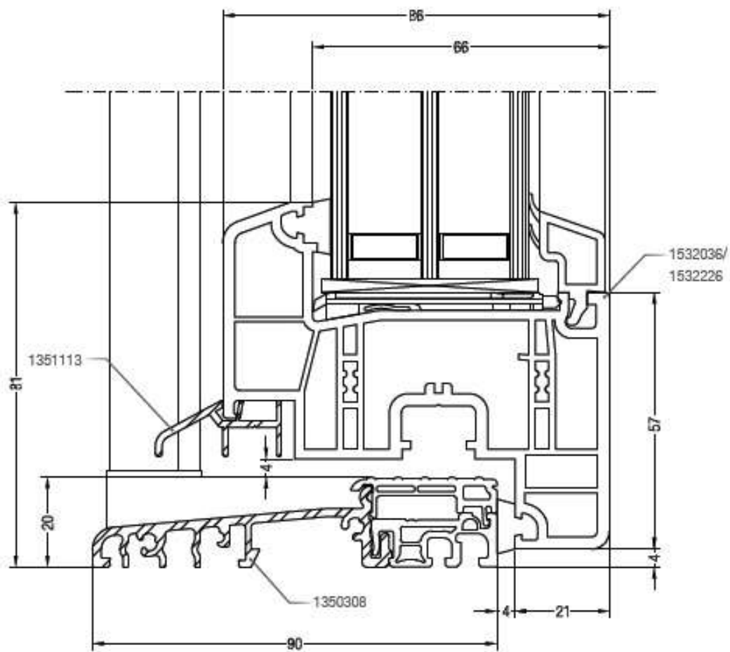
Sezione nodo anta dritta da 57 mm e soglia in Al
