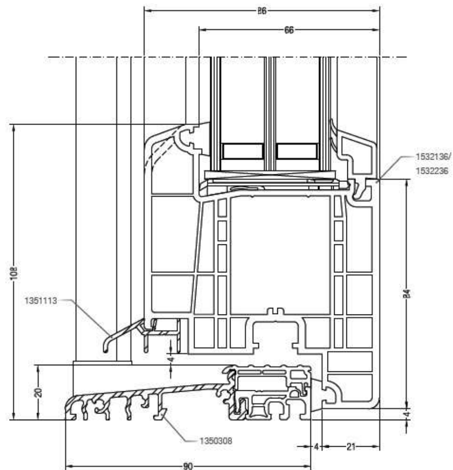
Sezione nodo anta dritta da 84 mm e soglia in Al
